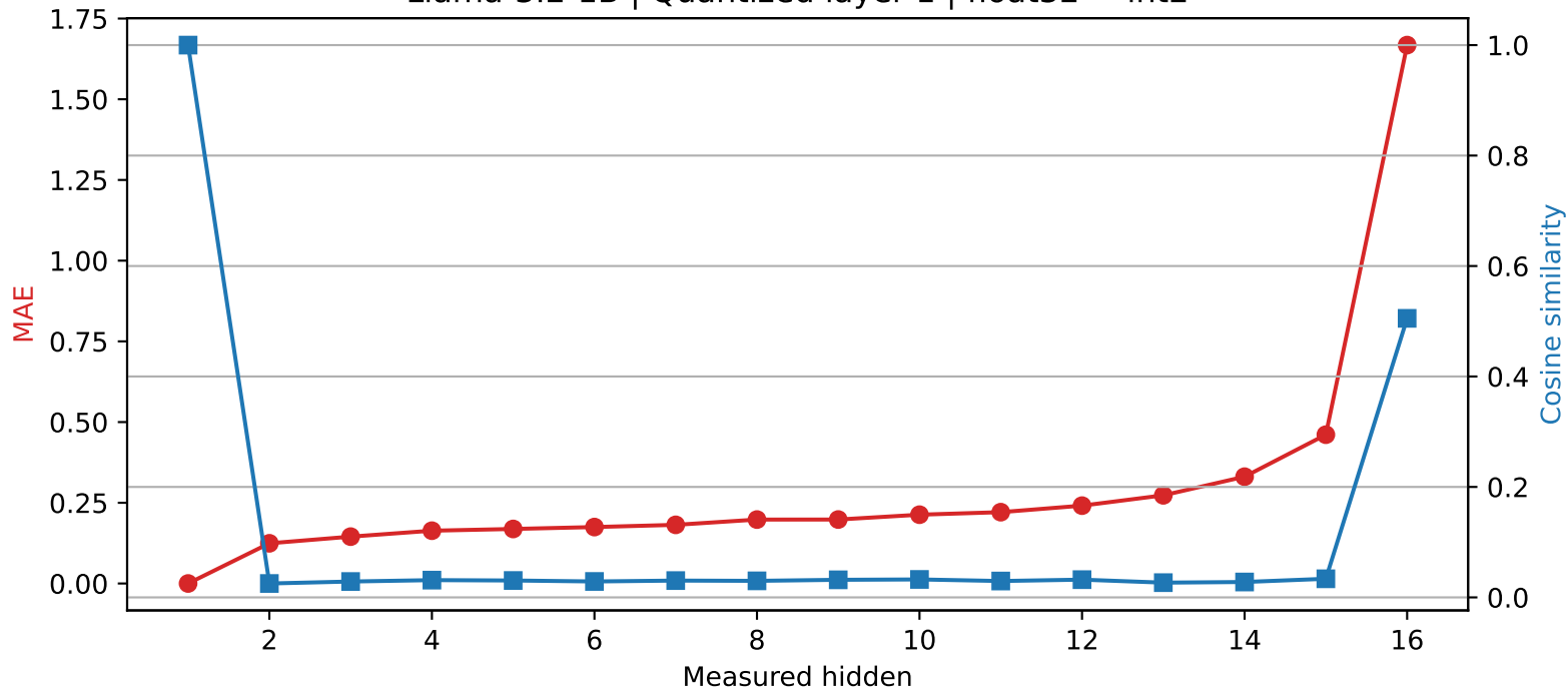
Llama-3.2-1B | Quantized layer 1 | float32 \rightarrow int2
