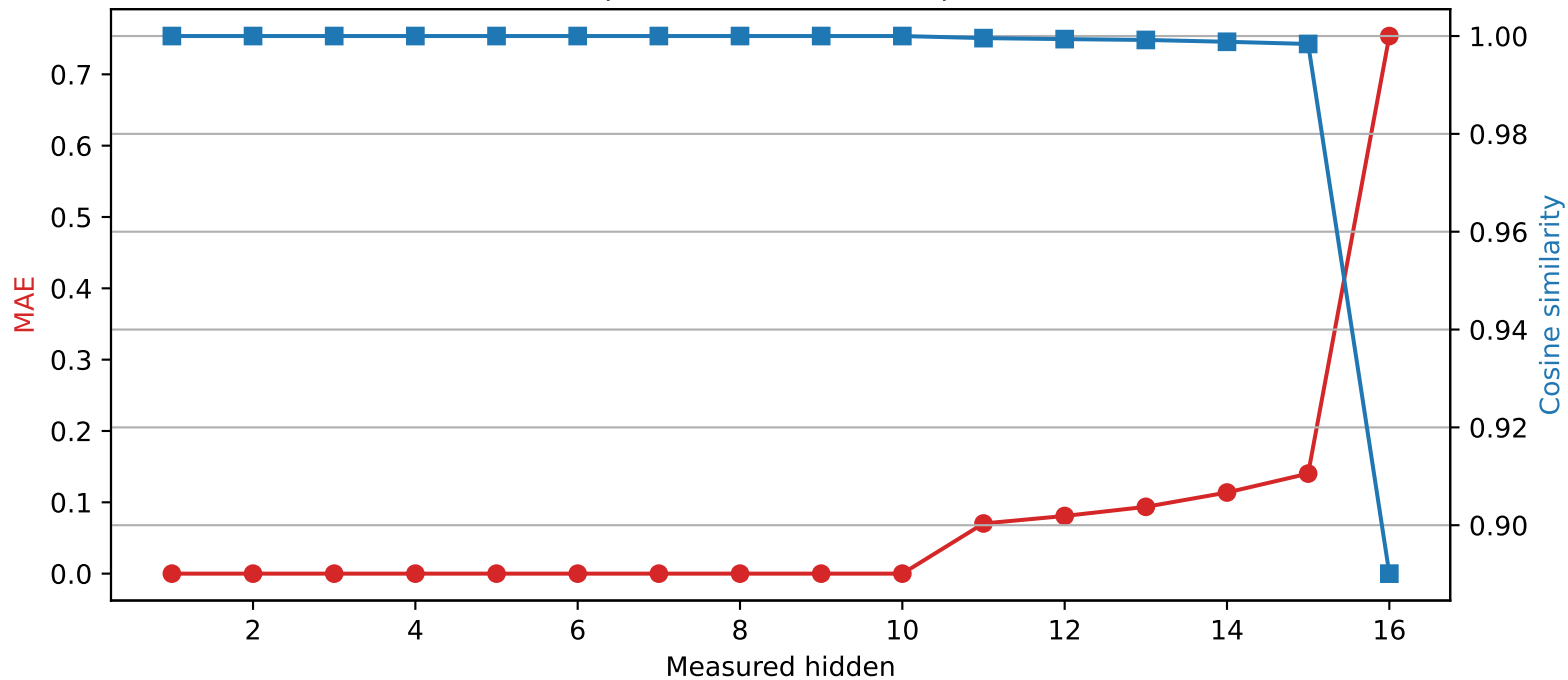
Llama-3.2-1B | Quantized layer 10 | float32 \rightarrow int2
