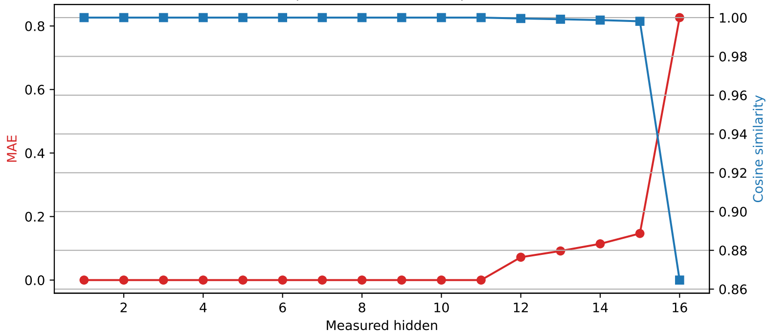
Llama-3.2-1B | Quantized layer 11 | float32 \rightarrow int2
