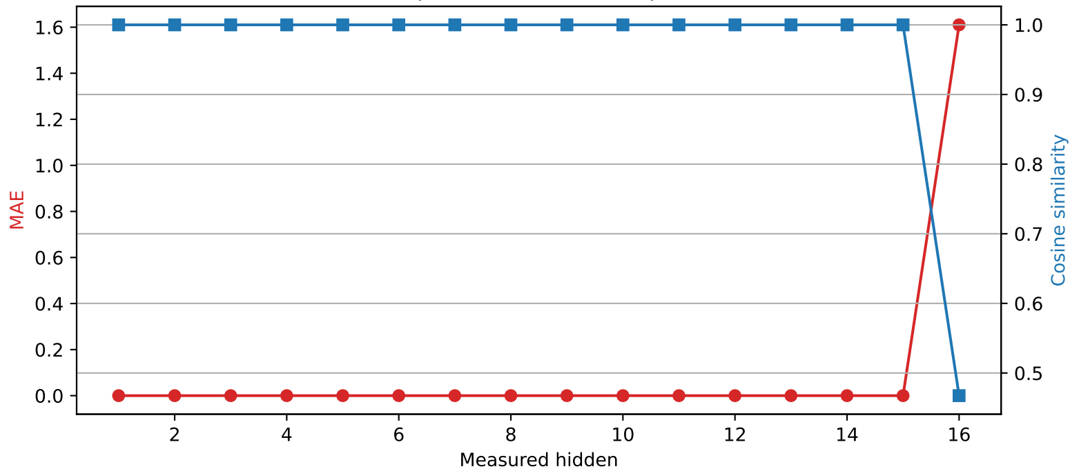
Llama-3.2-1B | Quantized layer 15 | float32 \rightarrow int2
