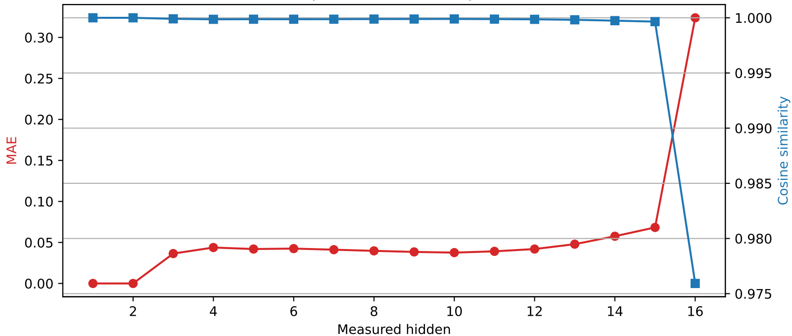
Llama-3.2-1B | Quantized layer 2 | float32 \rightarrow int2
