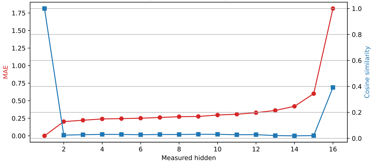
Llama-3.2-1B | Quantized layer 1 | float64 \rightarrow int2
