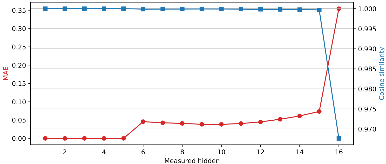
Llama-3.2-1B | Quantized layer 5 | float64 \rightarrow int2
