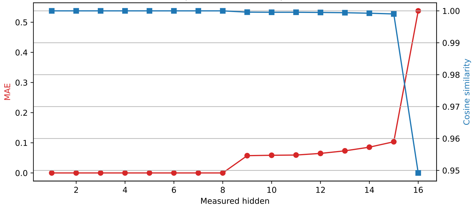
Llama-3.2-1B | Quantized layer 8 | float64 \rightarrow int2
