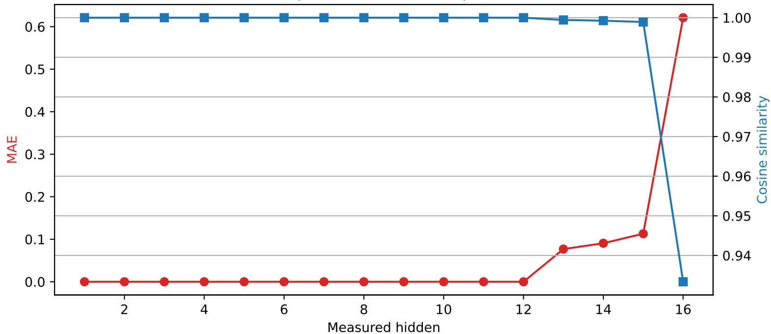
Llama-3.2-1B | Quantized layer 12 | float64 \rightarrow int2
