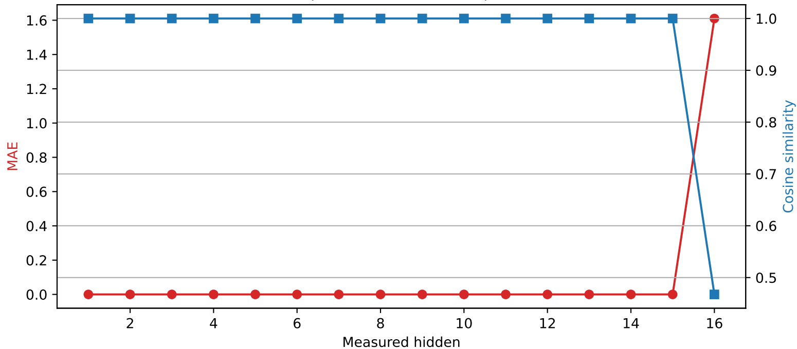
Llama-3.2-1B | Quantized layer 15 | float64 \rightarrow int2
