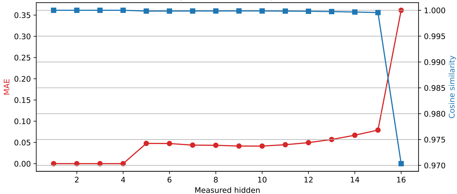
Llama-3.2-1B | Quantized layer 4 | float64 \rightarrow int2
