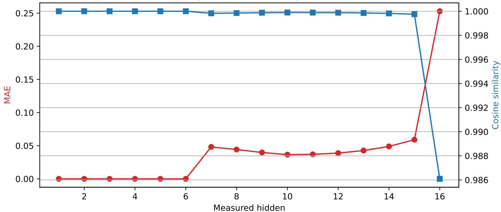
Llama-3.2-1B | Quantized layer 6 | float64 \rightarrow int2
