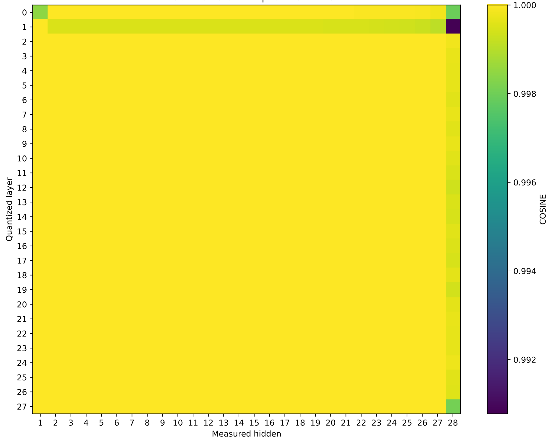
Model: Llama-3.2-3B | float16 \rightarrow int8
