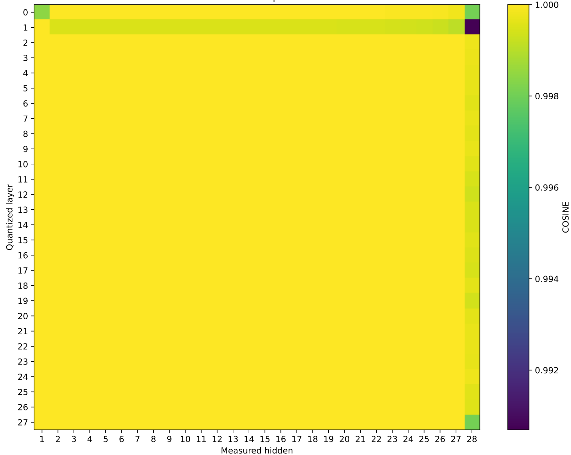
Model: Llama-3.2-3B | float32 \rightarrow int8
