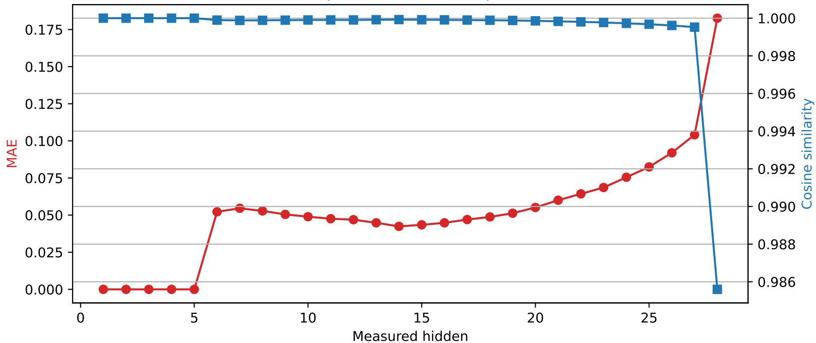
Llama-3.2-3B | Quantized layer 5 | float16 \rightarrow int4
