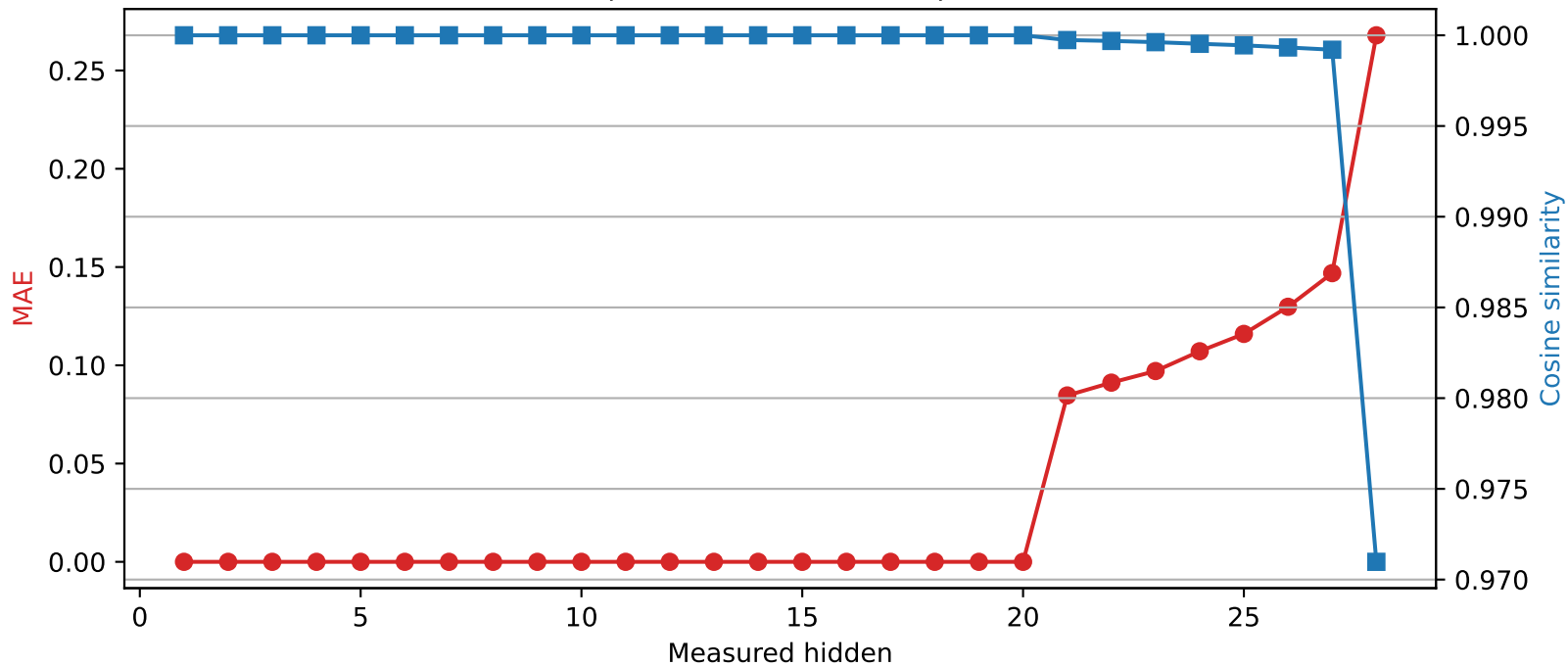
Llama-3.2-3B | Quantized layer 20 | float32 \rightarrow int4
