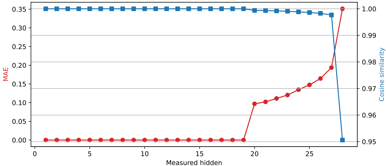
Llama-3.2-3B | Quantized layer 19 | float32 \rightarrow int4
