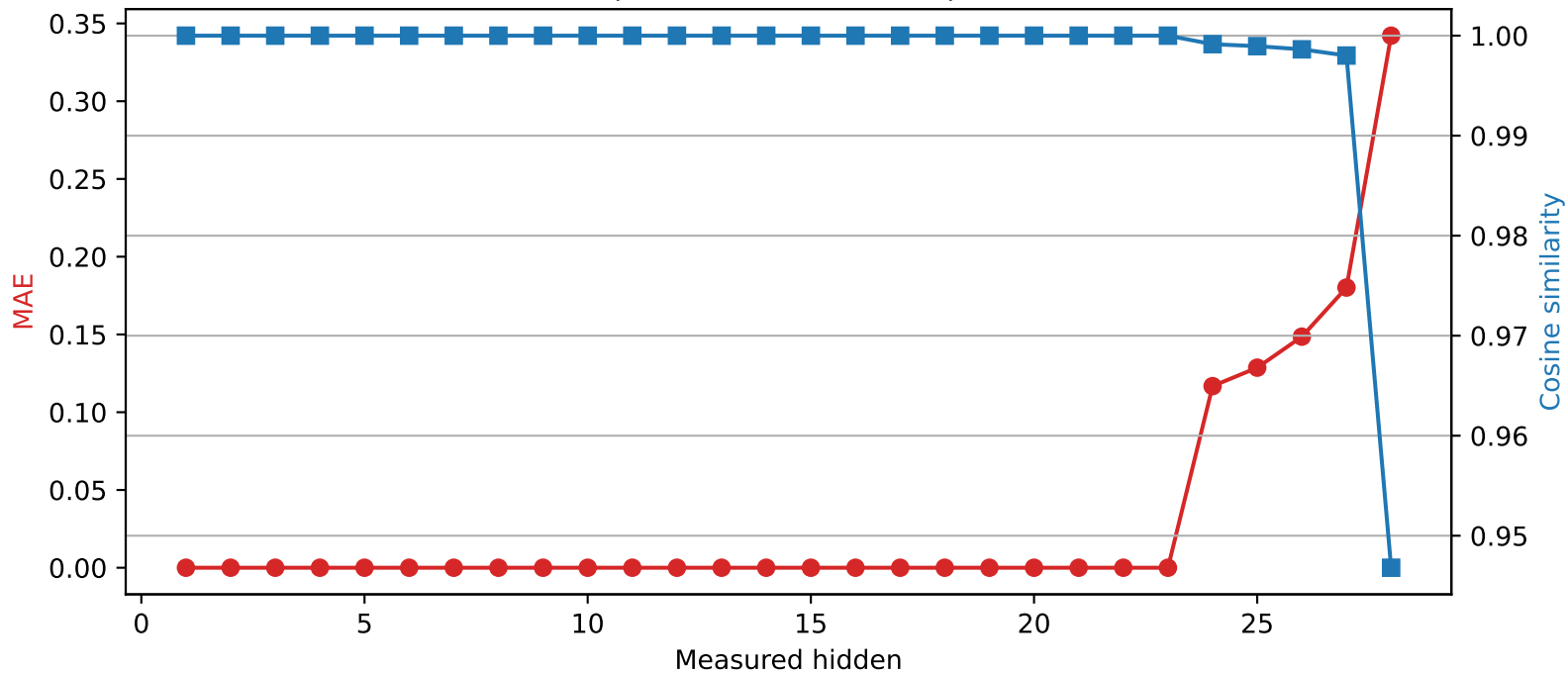
Llama-3.2-3B | Quantized layer 23 | float32 \rightarrow int4
