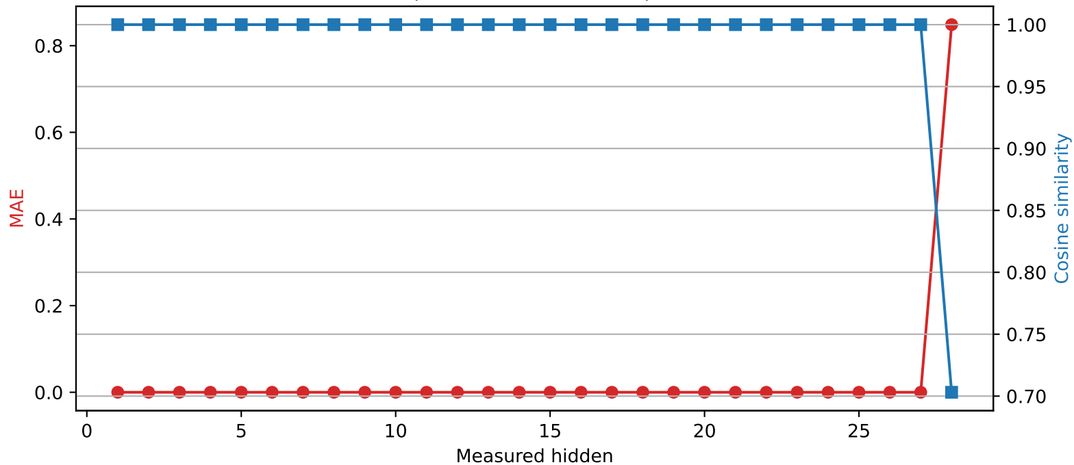
Llama-3.2-3B | Quantized layer 27 | float64 \rightarrow int4
