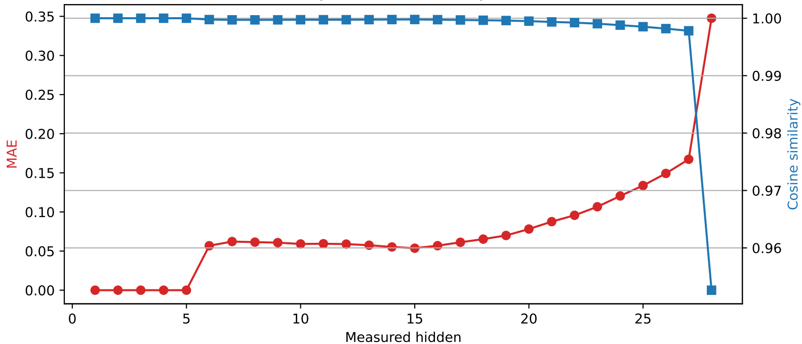
Llama-3.2-3B | Quantized layer 5 | float64 \rightarrow int4
