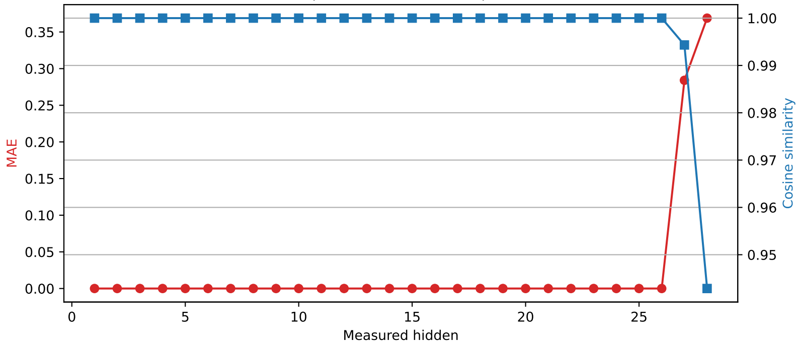
Llama-3.2-3B | Quantized layer 26 | float64 \rightarrow int4
