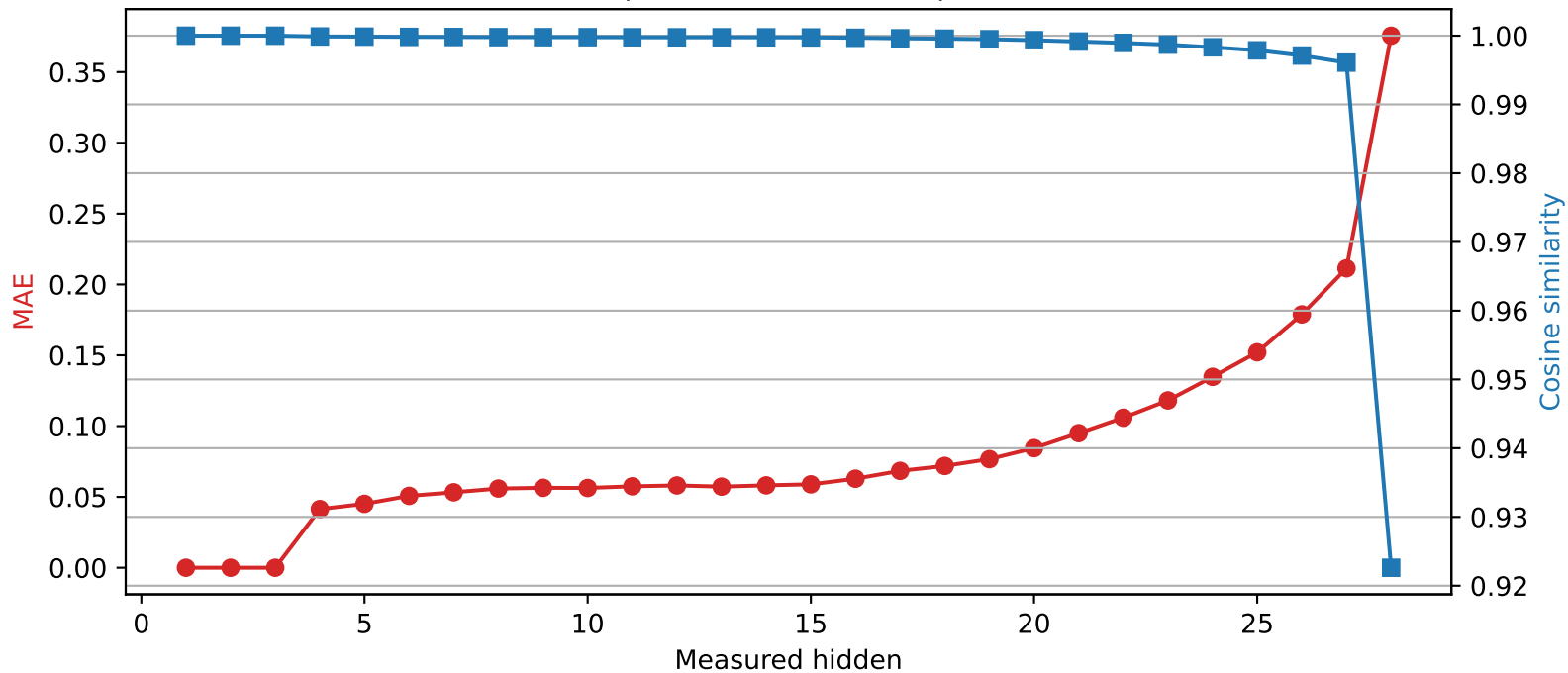
Llama-3.2-3B | Quantized layer 3 | float16 \rightarrow int2
