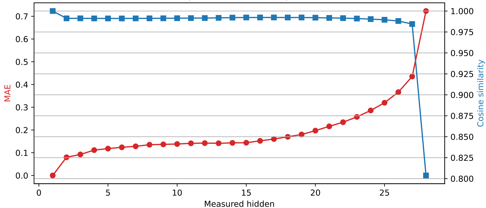
Llama-3.2-3B | Quantized layer 1 | float16 \rightarrow int2
