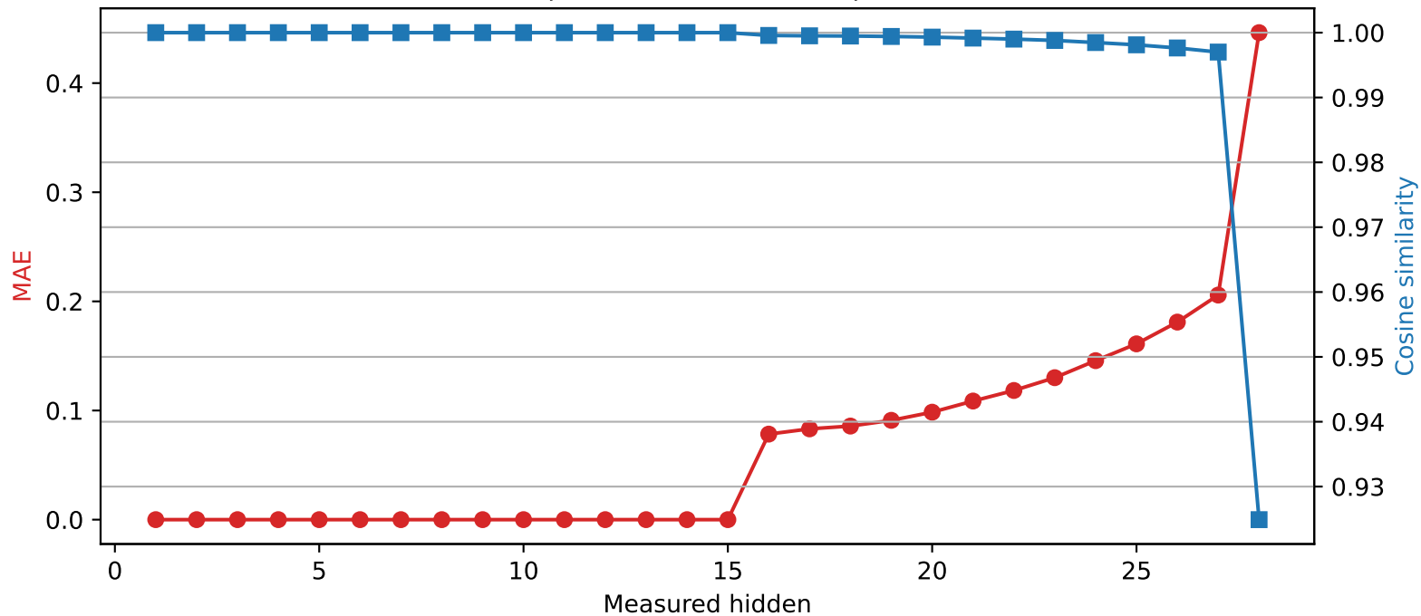
Llama-3.2-3B | Quantized layer 15 | float16 \rightarrow int2
