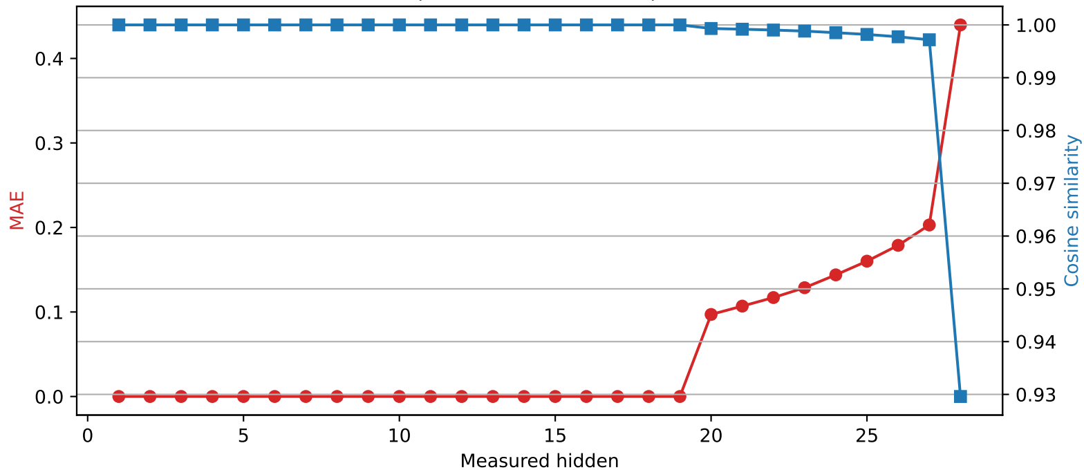
Llama-3.2-3B | Quantized layer 19 | float16 \rightarrow int2
