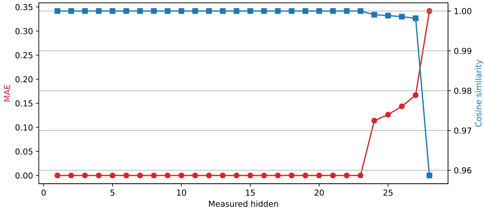
Llama-3.2-3B | Quantized layer 23 | float16 \rightarrow int2
