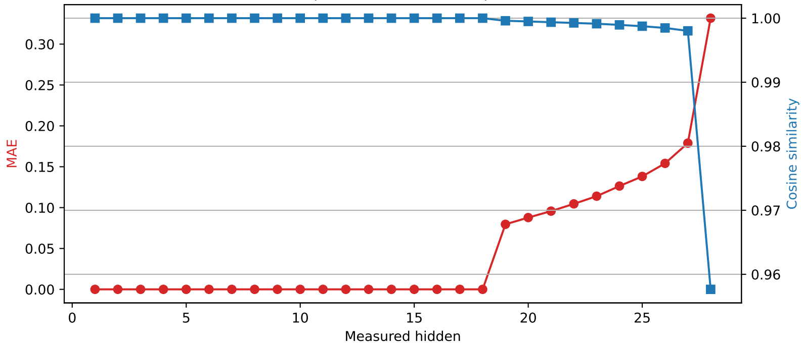
Llama-3.2-3B | Quantized layer 18 | float16 \rightarrow int2
