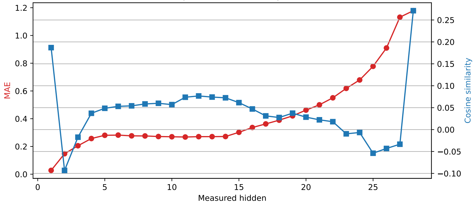
Llama-3.2-3B | Quantized layer 0 | float16 \rightarrow int2
