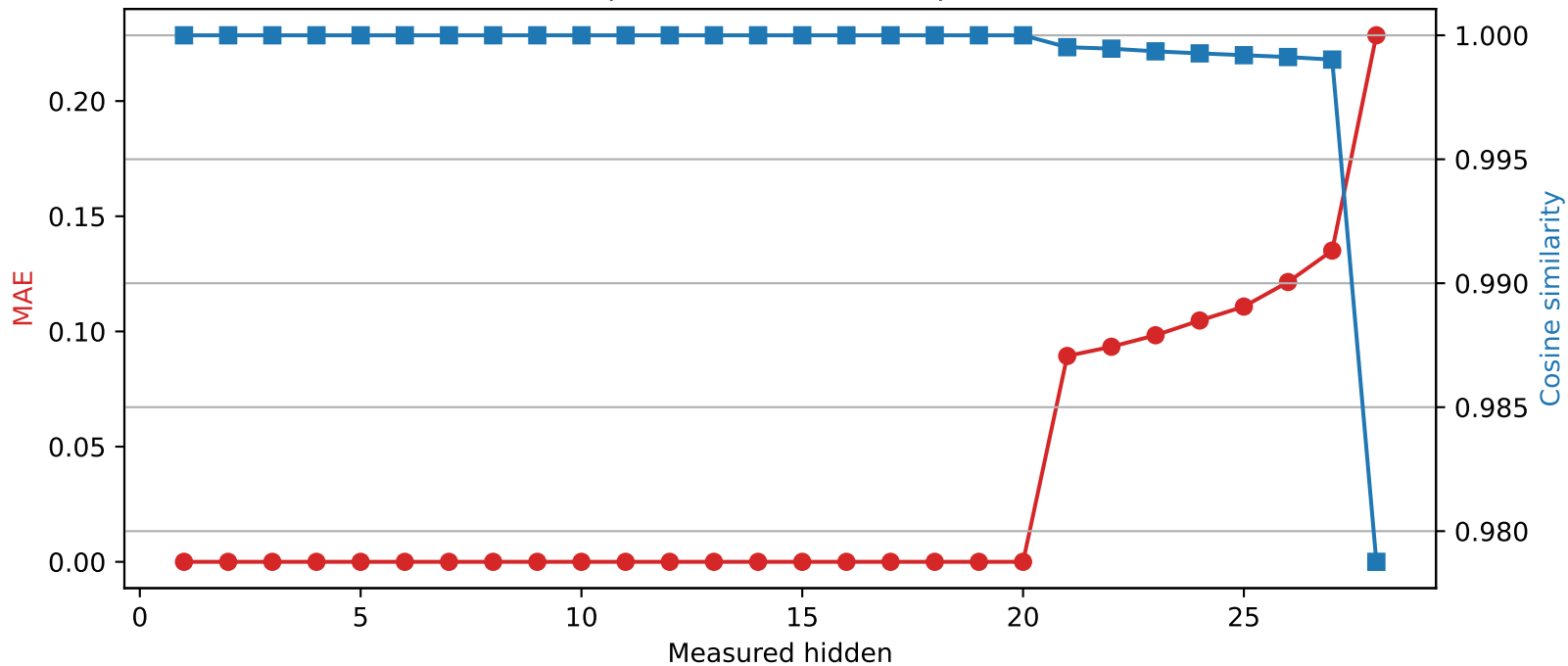
Llama-3.2-3B | Quantized layer 20 | float16 \rightarrow int2
