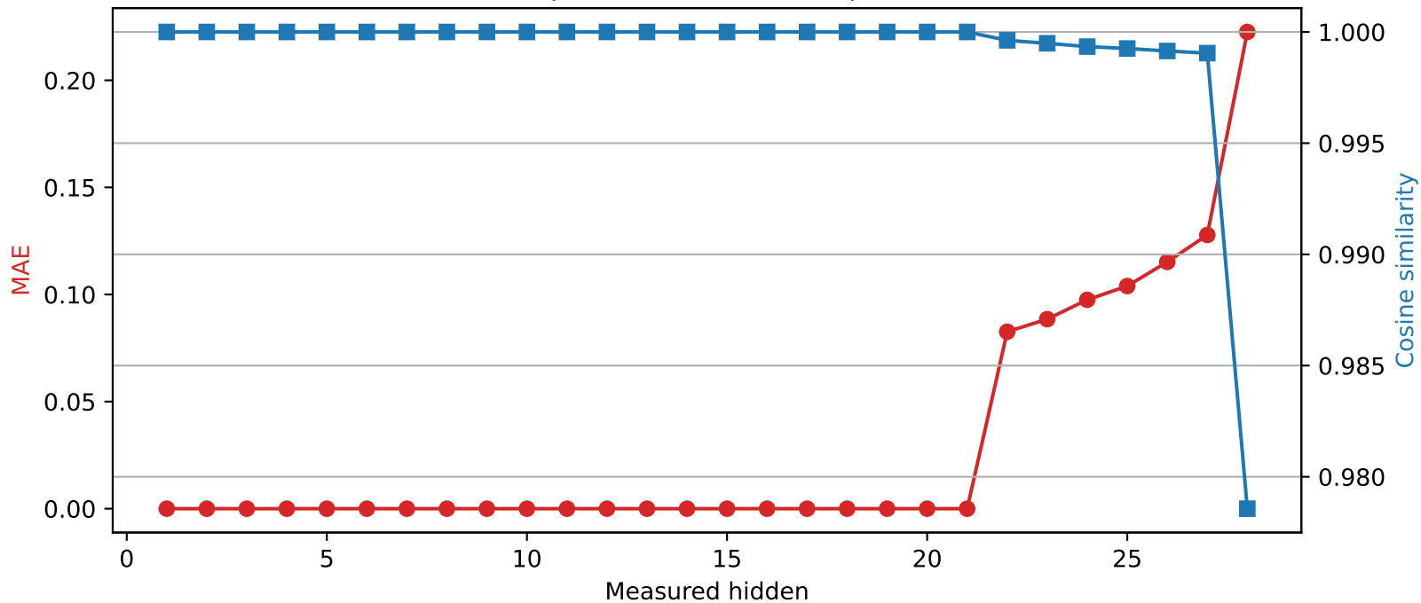
Llama-3.2-3B | Quantized layer 21 | float16 \rightarrow int2
