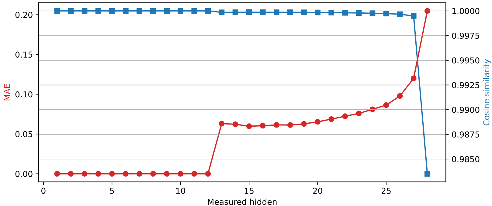
Llama-3.2-3B | Quantized layer 12 | float32 \rightarrow int2
