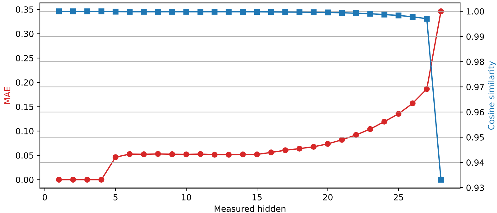
Llama-3.2-3B | Quantized layer 4 | float32 \rightarrow int2
