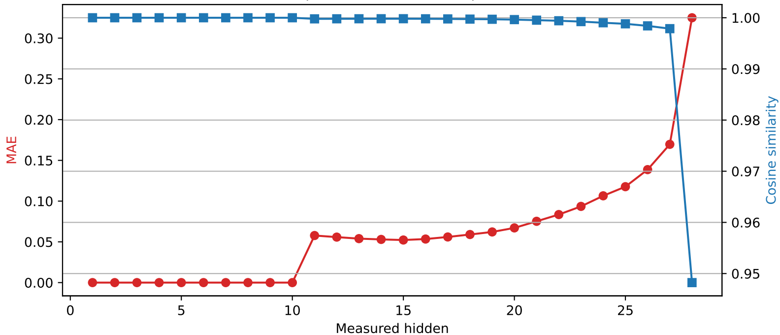
Llama-3.2-3B | Quantized layer 10 | float32 \rightarrow int2
