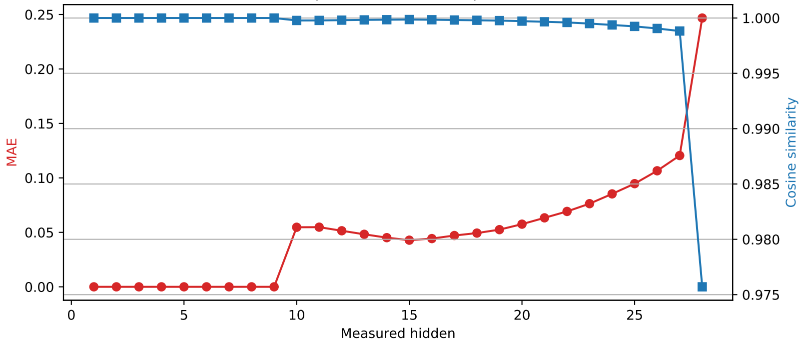
Llama-3.2-3B | Quantized layer 9 | float32 \rightarrow int2
