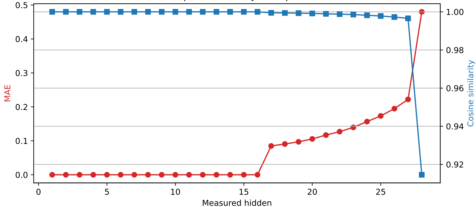
Llama-3.2-3B | Quantized layer 16 | float32 \rightarrow int2
