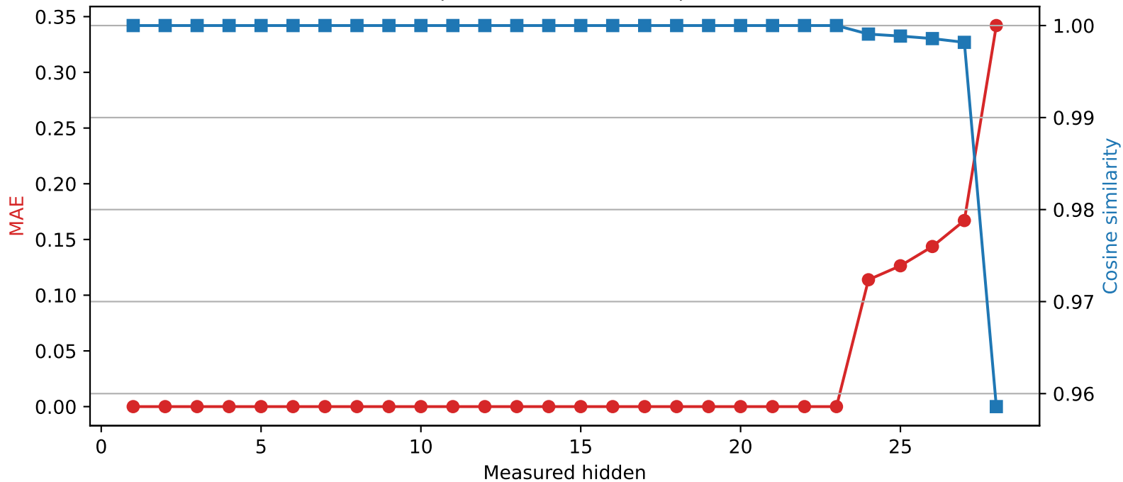
Llama-3.2-3B | Quantized layer 23 | float32 \rightarrow int2
