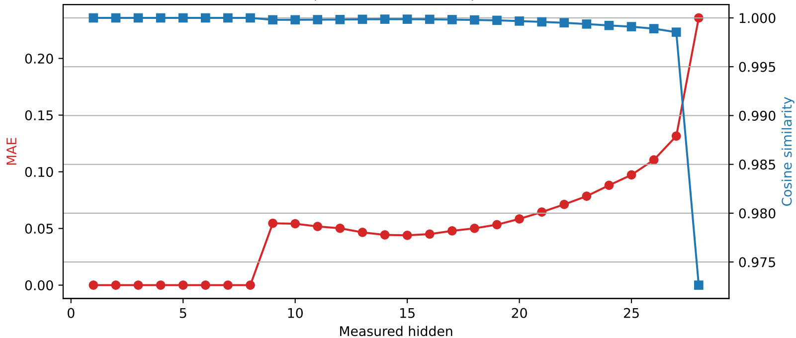
Llama-3.2-3B | Quantized layer 8 | float32 \rightarrow int2
