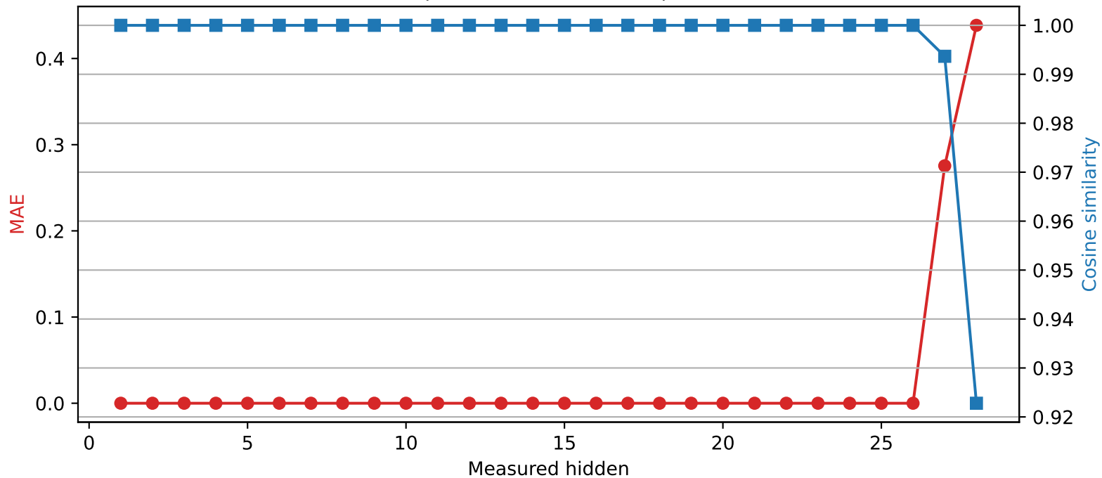
Llama-3.2-3B | Quantized layer 26 | float32 \rightarrow int2
