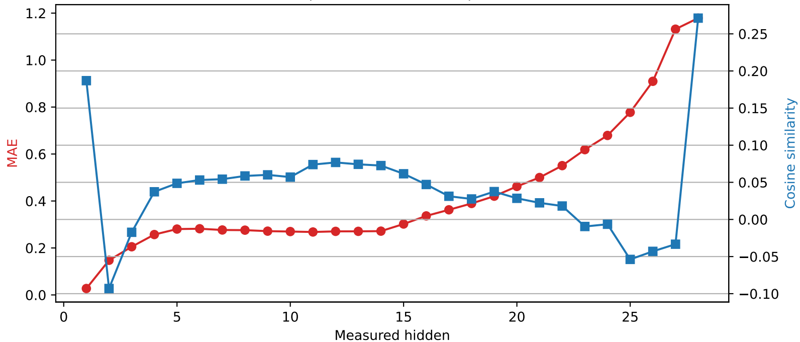
Llama-3.2-3B | Quantized layer 0 | float32 \rightarrow int2
