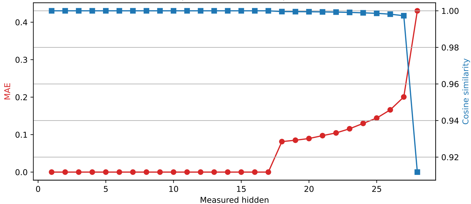
Llama-3.2-3B | Quantized layer 17 | float64 \rightarrow int2
