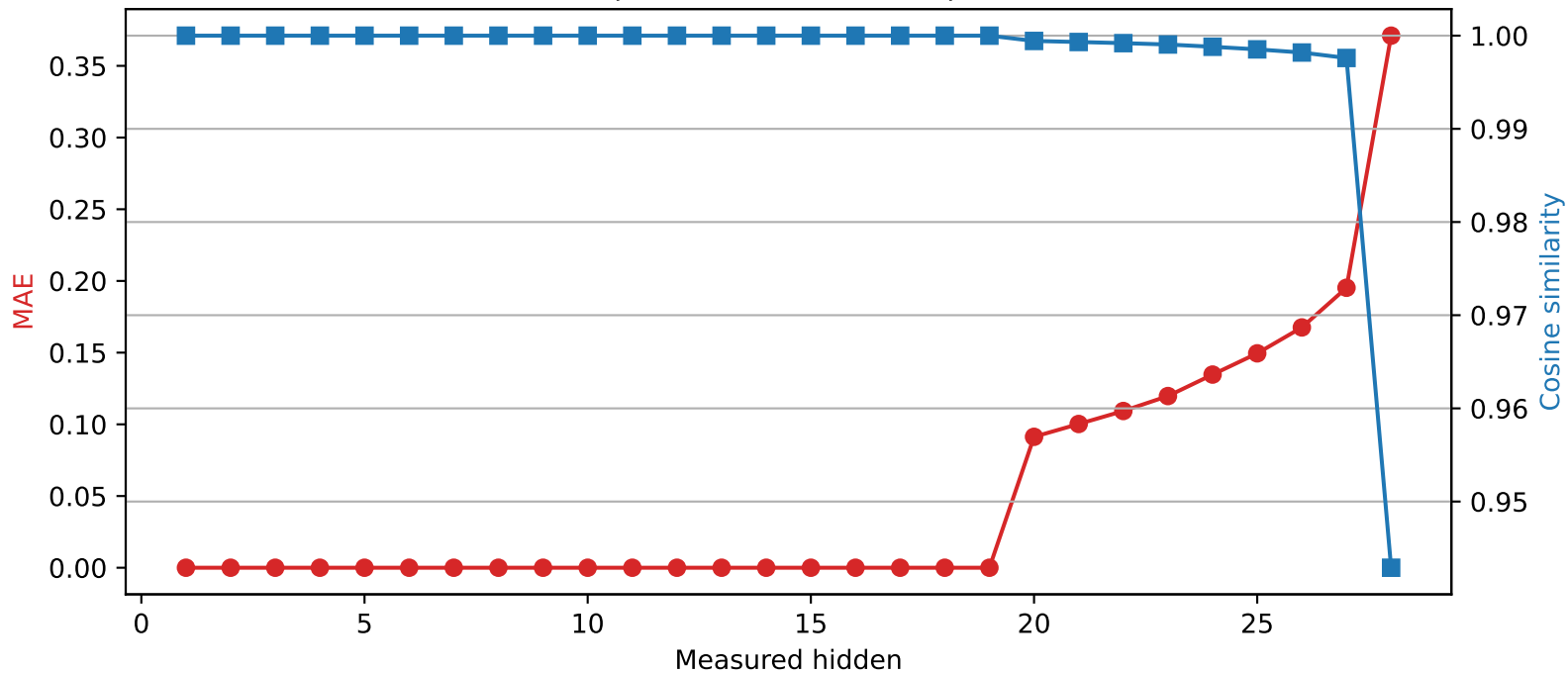
Llama-3.2-3B | Quantized layer 19 | float64 \rightarrow int2
