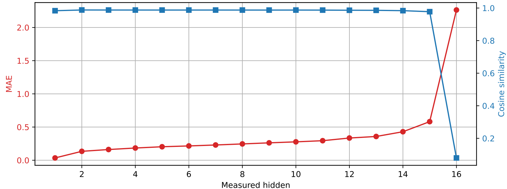
Llama-3.2-1B | Prompt 0 Spared layer 11 | Unquantized vs hybrid
