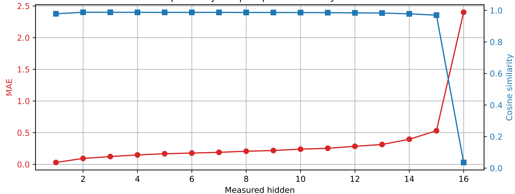
Llama-3.2-1B | Prompt 1 Spared layer 8 | Unquantized vs hybrid
