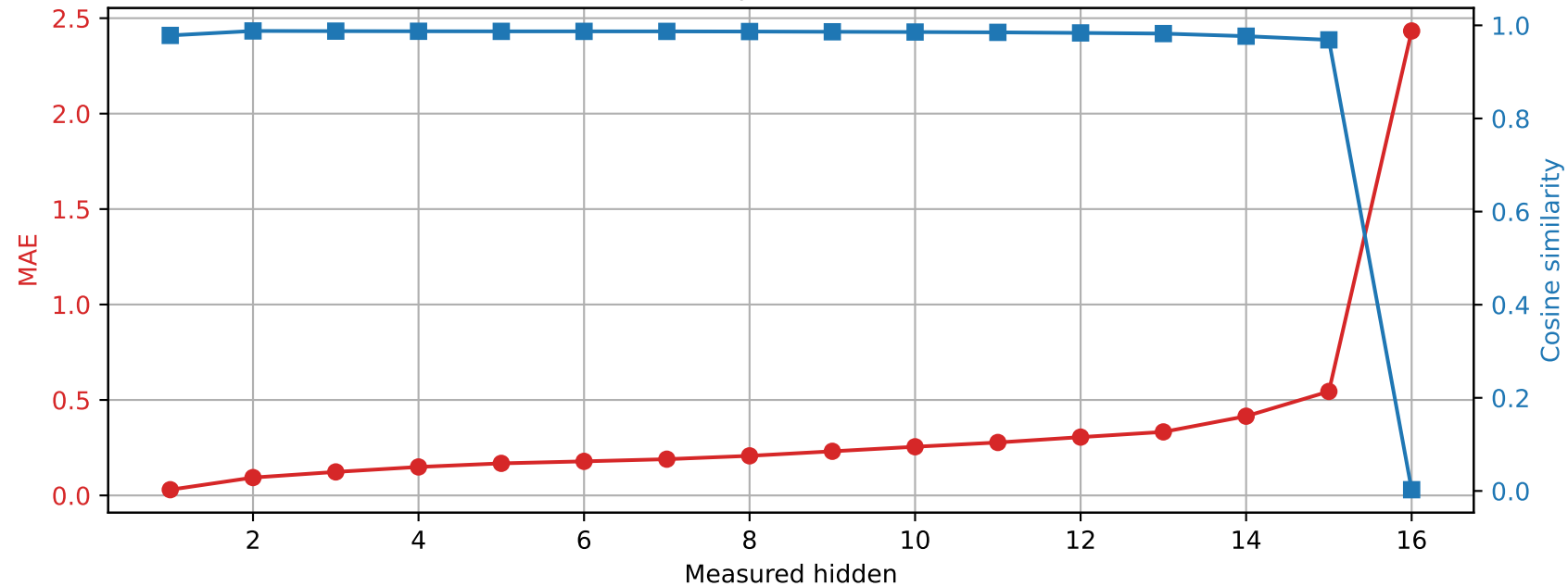
Llama-3.2-1B | Prompt 1 Spared layer 10 | Unquantized vs hybrid
