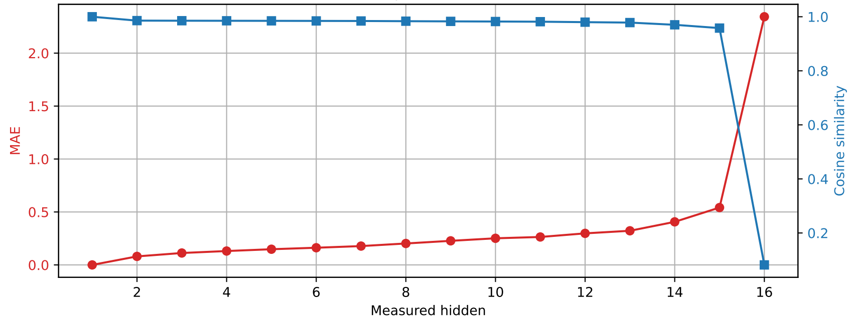
Llama-3.2-1B | Prompt 2 Spared layer 0 | Unquantized vs hybrid
