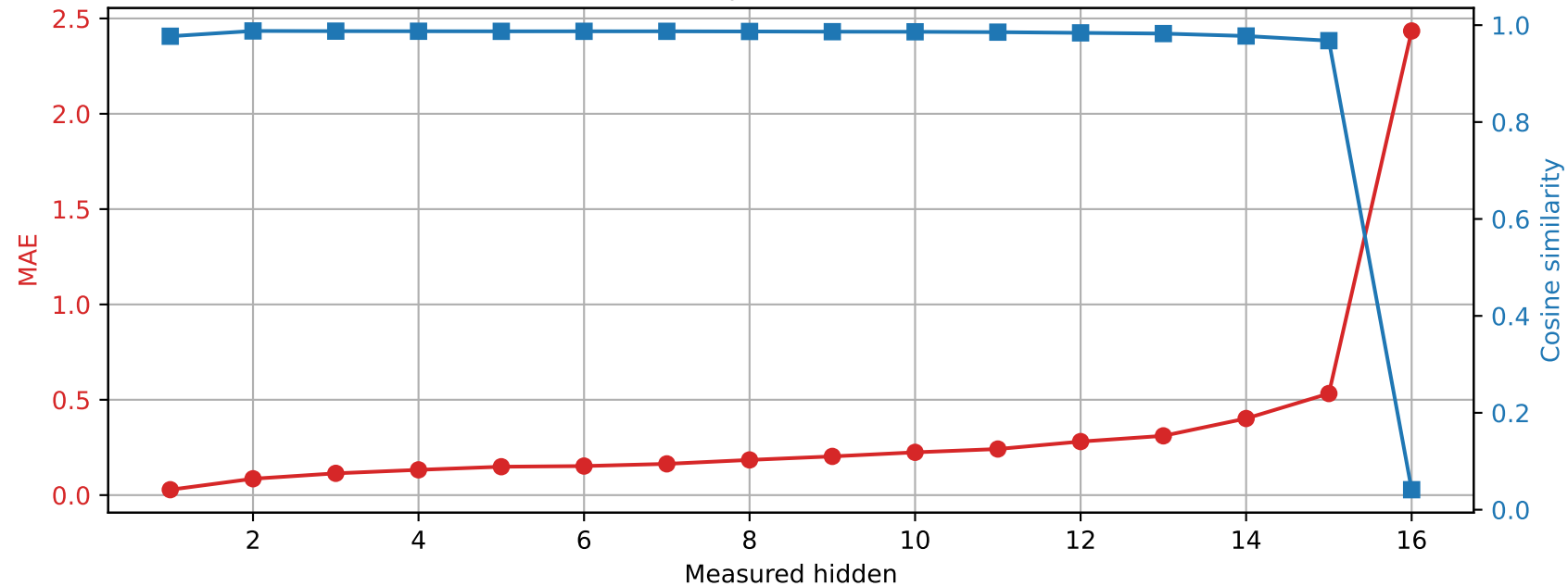
Llama-3.2-1B | Prompt 2 Spared layer 5 | Unquantized vs hybrid
