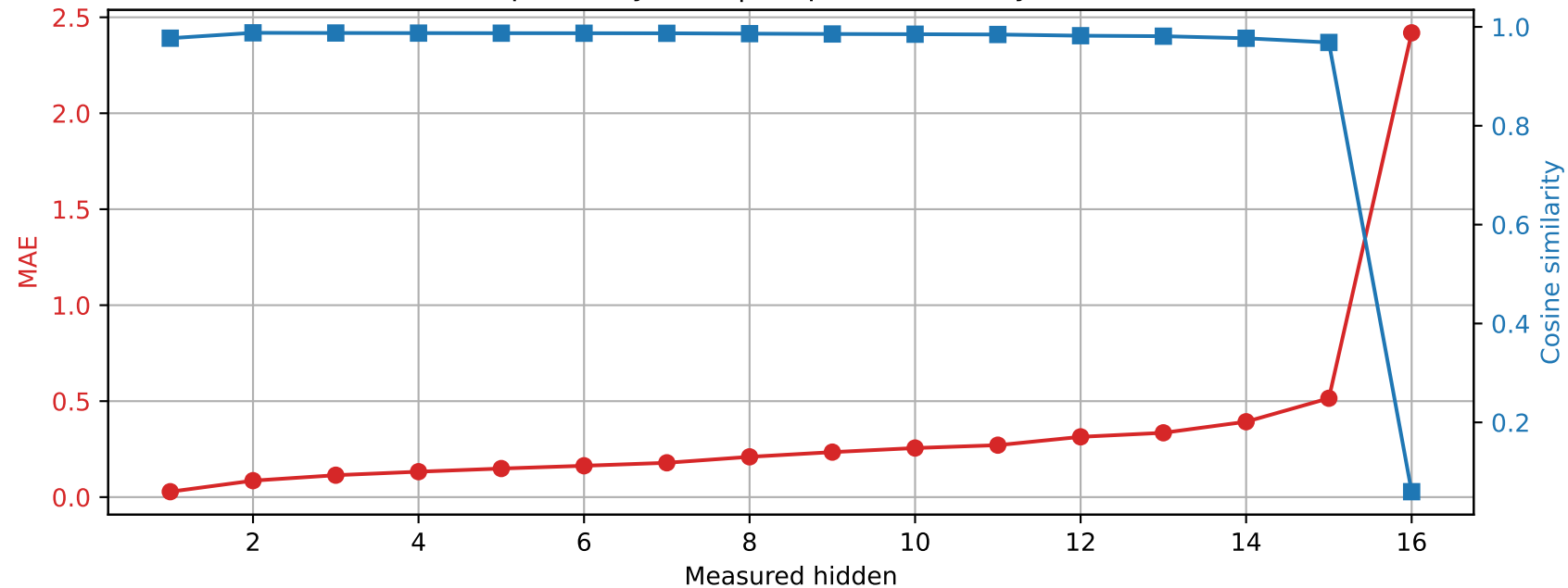
Llama-3.2-1B | Prompt 2 Spared layer 11 | Unquantized vs hybrid
