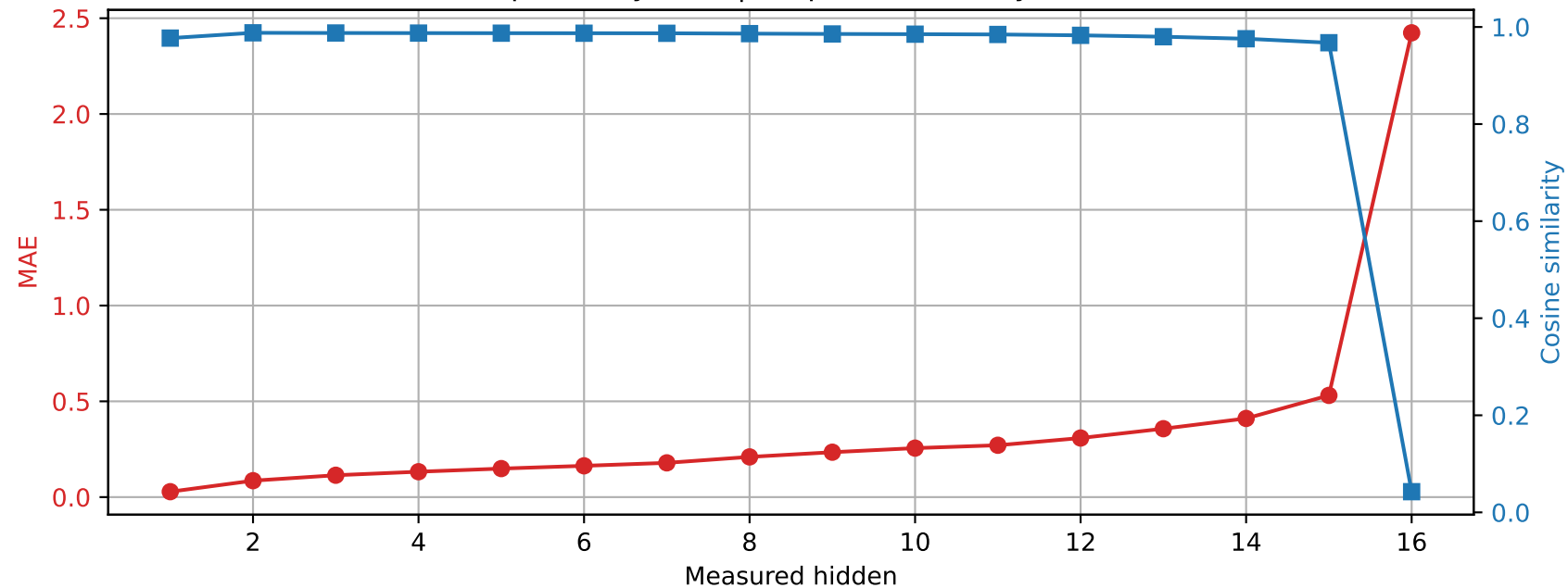
Llama-3.2-1B | Prompt 2 Spared layer 12 | Unquantized vs hybrid
