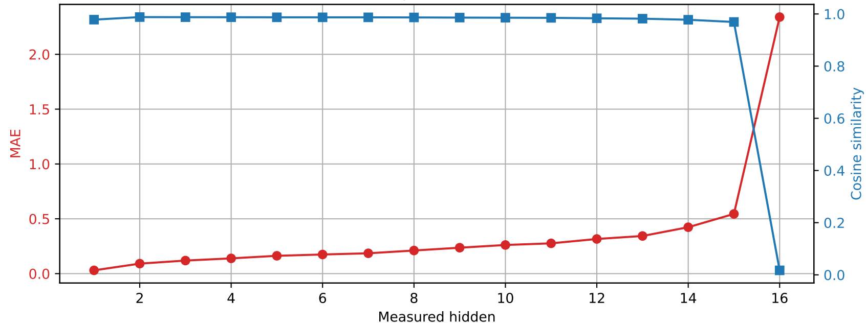
Llama-3.2-1B | Prompt 3 Spared layer 5 | Unquantized vs hybrid
