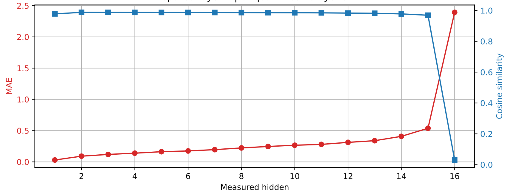
Llama-3.2-1B | Prompt 3 Spared layer 7 | Unquantized vs hybrid
